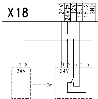
Nadajnik Bramka świetlna jednowiązkowa pojedyncza, jako zabezpieczenie przed wciągnięciem podle EN 12978
