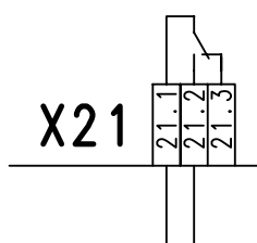
Kontakt przełącznikowy pozbawiony potencjału
