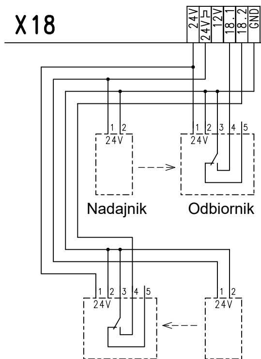
Odbiornik Bramka świetlna jednowiązkowa podwójna, jako zabezpieczenie przed wciągnięciem podle EN 12978
