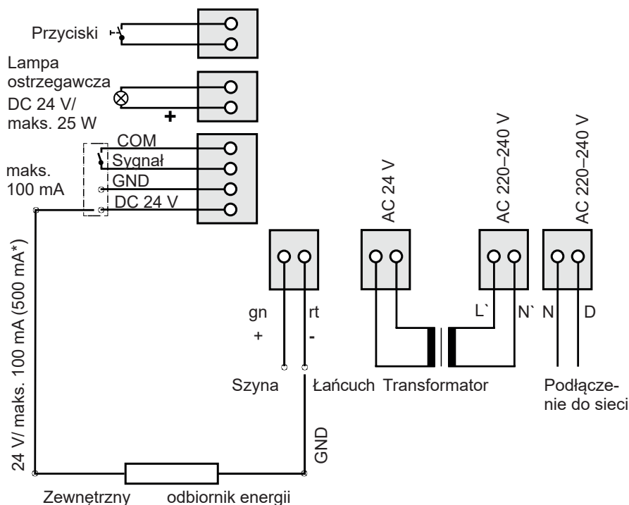
Rys. Schemat elektryczny sterownika stropowego
