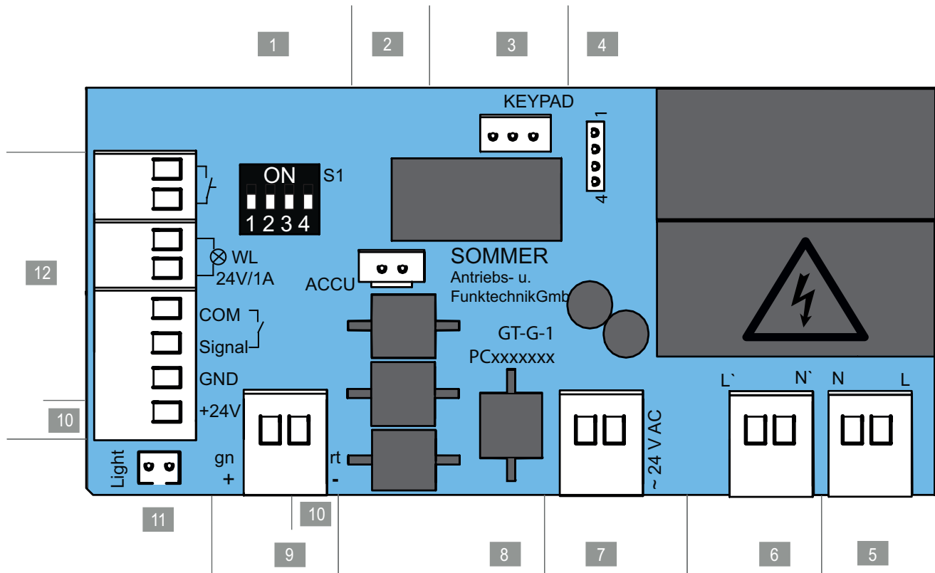
Rys. Płytki z obwodem drukowanym wózka jeźdnego, wersja pełna*
