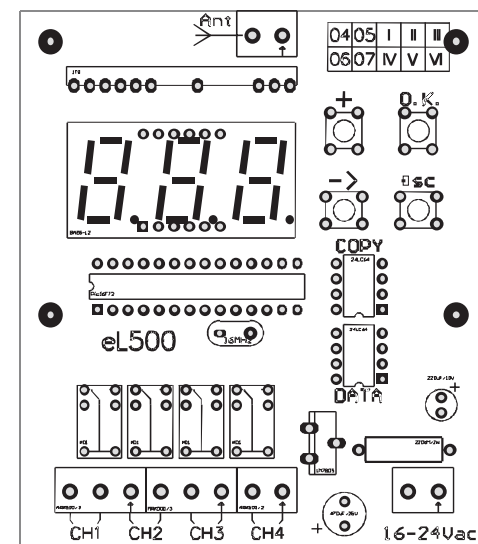
Widok od strony górnej
